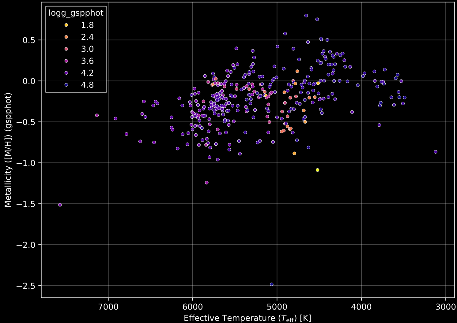
APOGEE DR17 Field: [266+64_btx] Stellar Population Parameters (n= 344)
